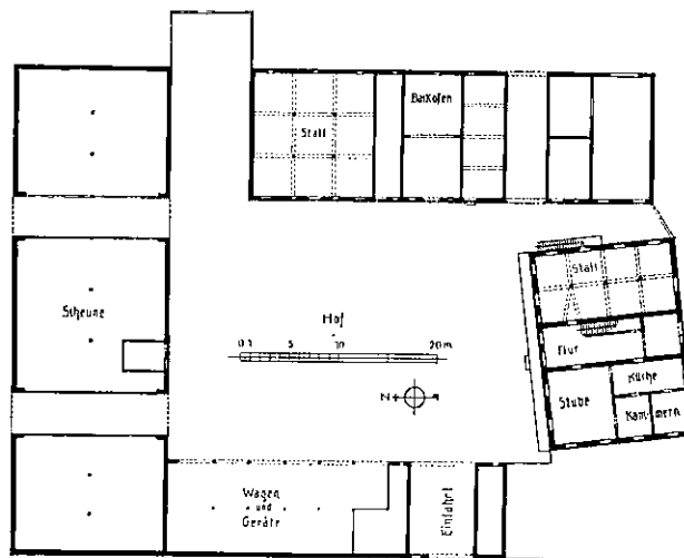
Grundriß eines Bauernhofes zu Vierhöfen, s. KDMNb 14, S. 329, Figur 267. Die stattlichen Gebäude sind heute abgerissen und durch gesichtslose Vorstadthaustypen ersetzt.
